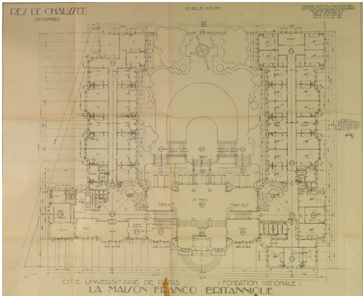
Plan du rez-de-chaussée, dressé par les architectes Pierre Martin et Maurice Vieu le 20 octobre 1932 et modifié les 20 mars et 10 mai 1933. Plan. Archives nationales, 20090013/333.
