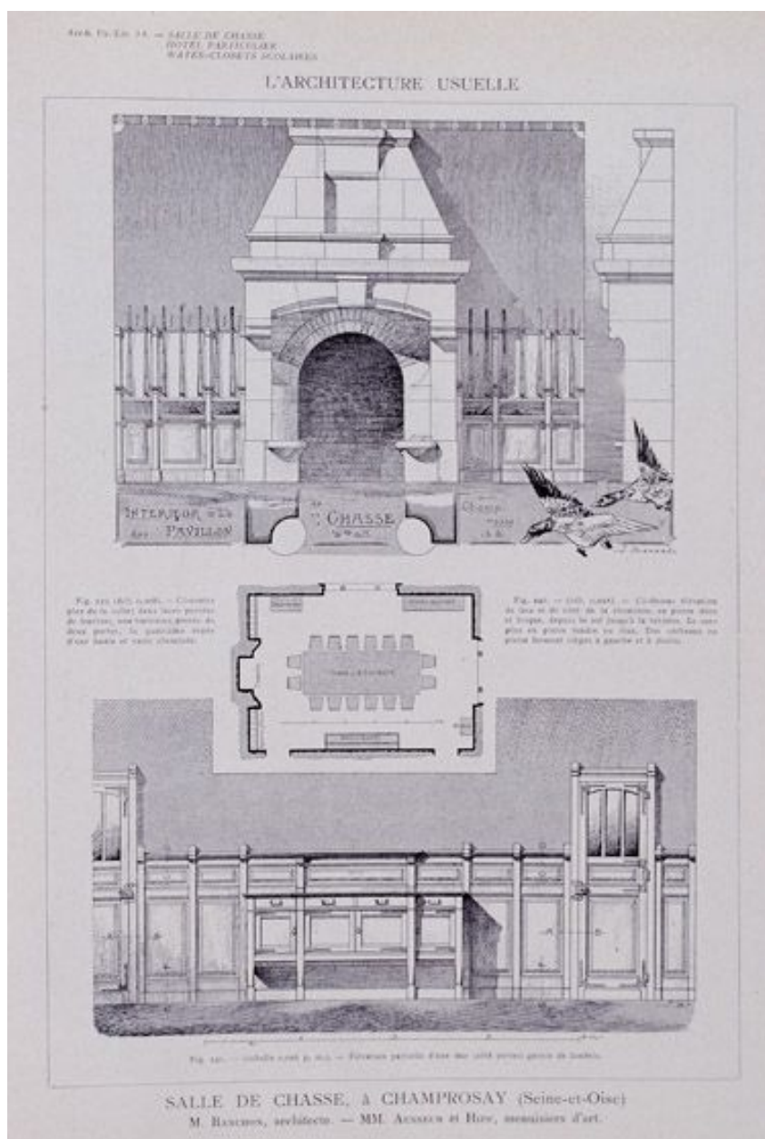
Salle de chasse située dans les communs : plan de la salle, élévation de la cheminée et élévation partielle d'une face garnie de lambris. Tiré de : L'Architecture usuelle, 1907. (BHVP, Per F° 537)
