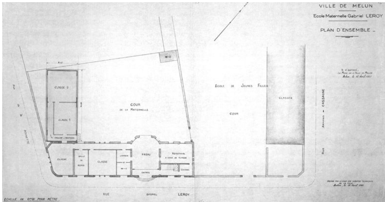
Plan de l'école maternelle Gabriel-Leroy. Tirage d'architecte, 1951. (AM Melun. 1 Fi 55)
