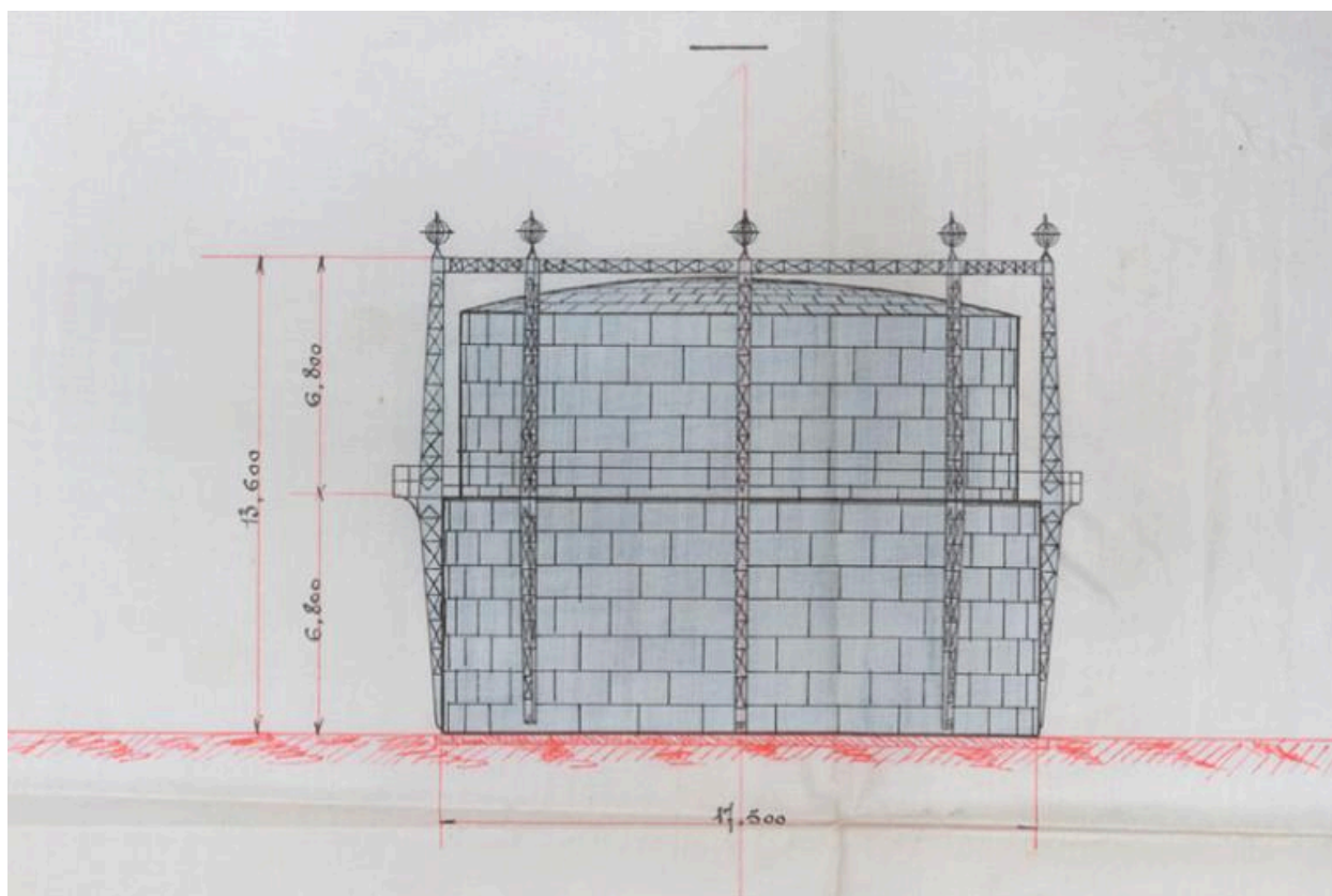
Elévation du gazomètre projeté en 1901. AM Mantes-la-Jolie, 4 O 13.
