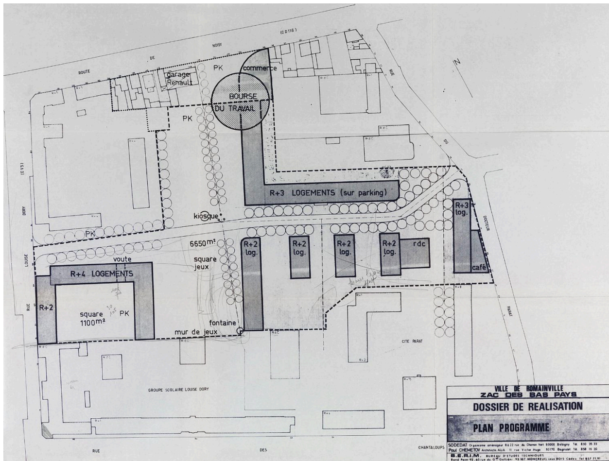
Z.A.C. des Bas-Pays. Plan masse. Architecte : Paul Chemetov. (AM Romainville)
