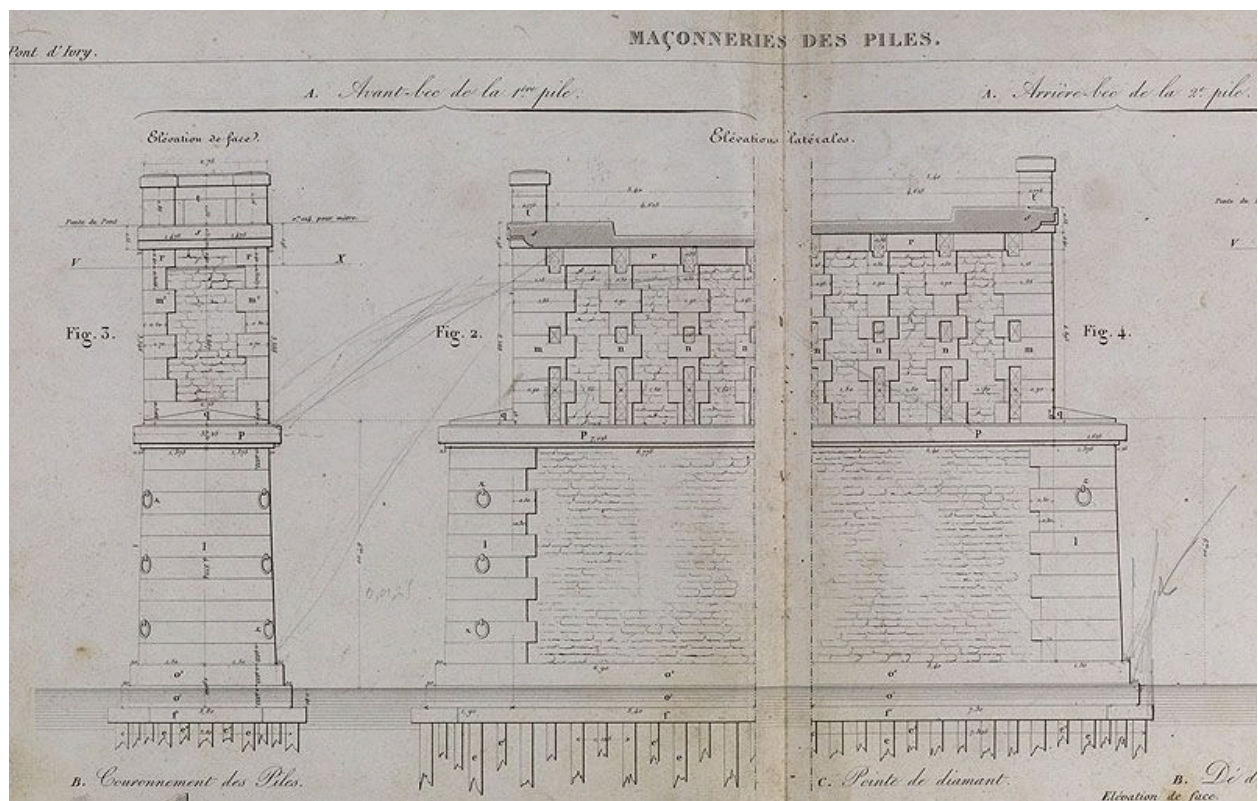
Ivry-sur-Seine. Pont d'Ivry (n°1). Elévations d'une pile. Tiré de : Pont d'Ivry en bois, sur piles en pierre, traversant la Seine... / MHC Emmery. Paris : Carilian-Goeyry, 1832. (Ecole nationale des ponts et chaussées)
