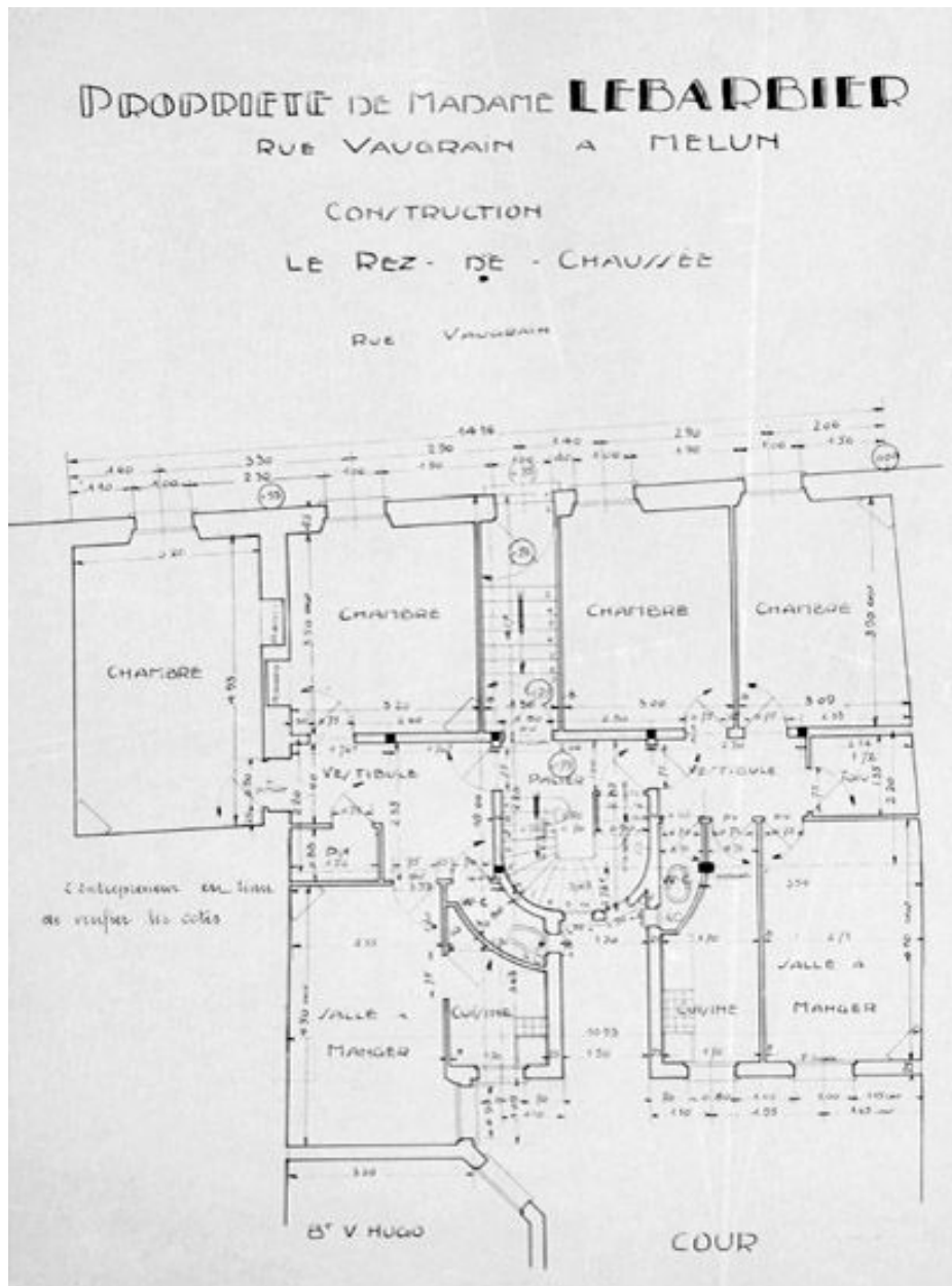
Immeuble, propriété de Mme Lebarbier, 1bis rue Vaugrain : plan du rez-de-chaussée. Tirage d'architecte, 1929-1930. (AM Melun. 1 Fi 961)
