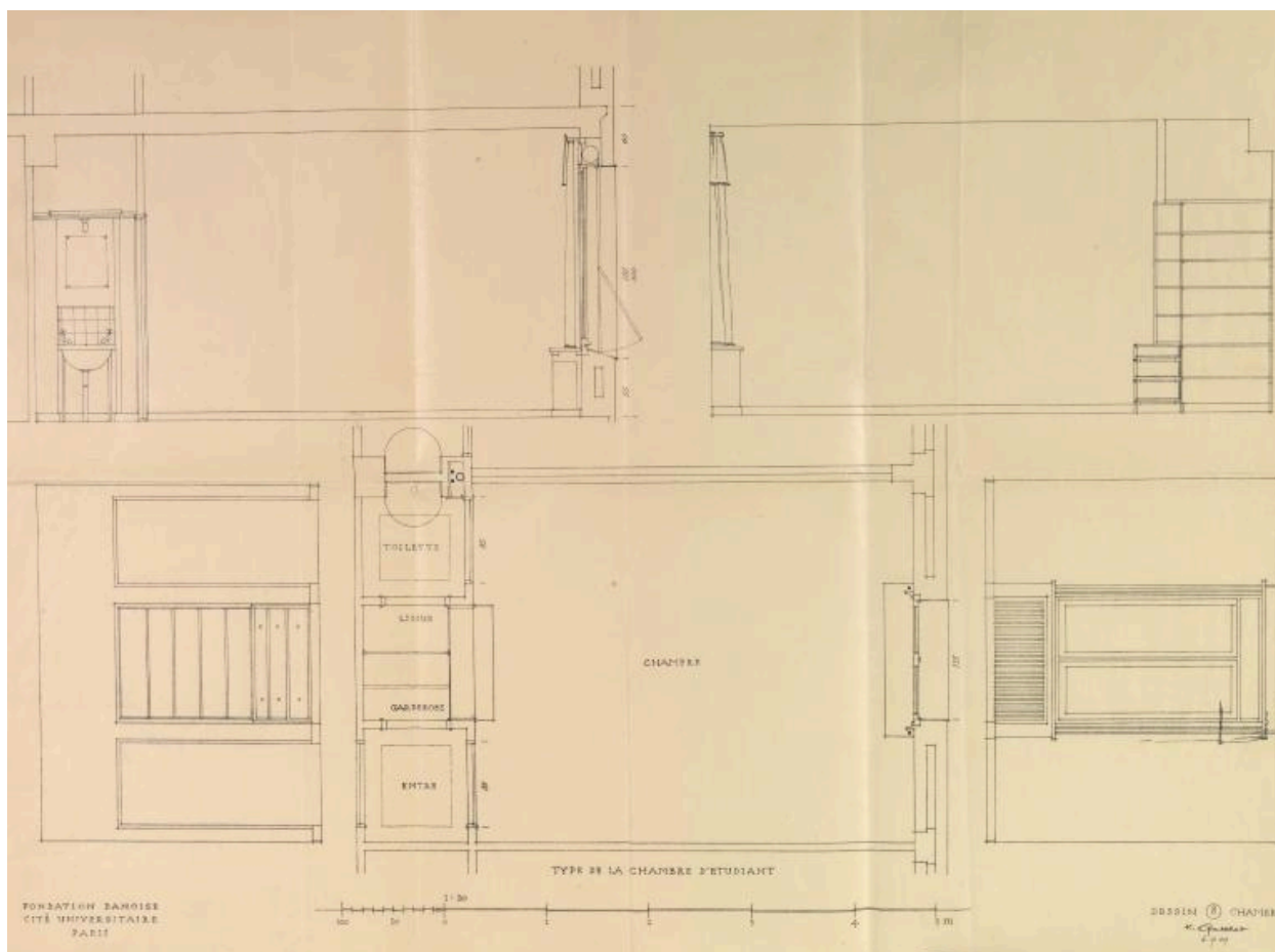
Schéma d'une chambre type ; dessin par K. Gottlob, architecte, 6 septembre 1929. Archives nationales, 20090013/374.
