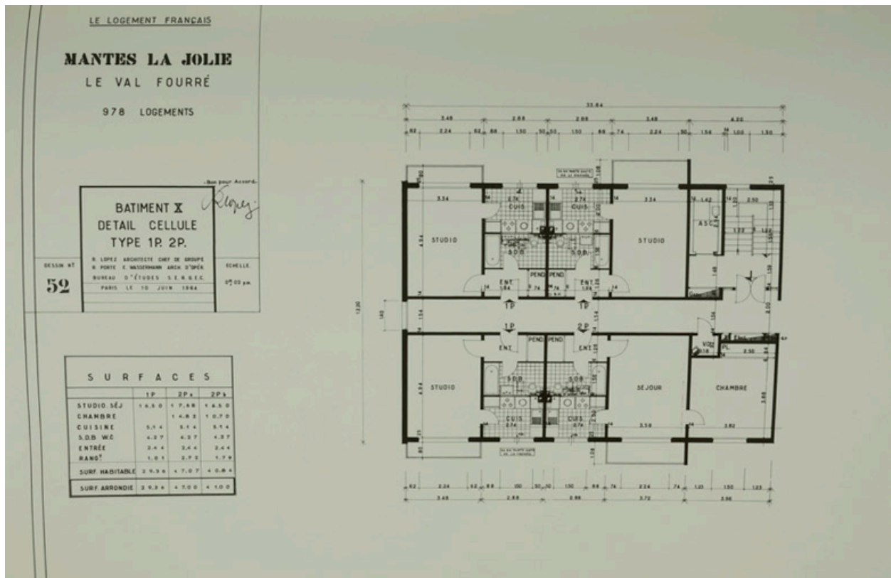
Quartier 1, des Ecrivains. Plan du bâtiment X de deux étages, cellules 1 pièce et 2 pièces. (Archives Nationales, Direction de l'Habitat et de la Construction, 19840091/58-59)
