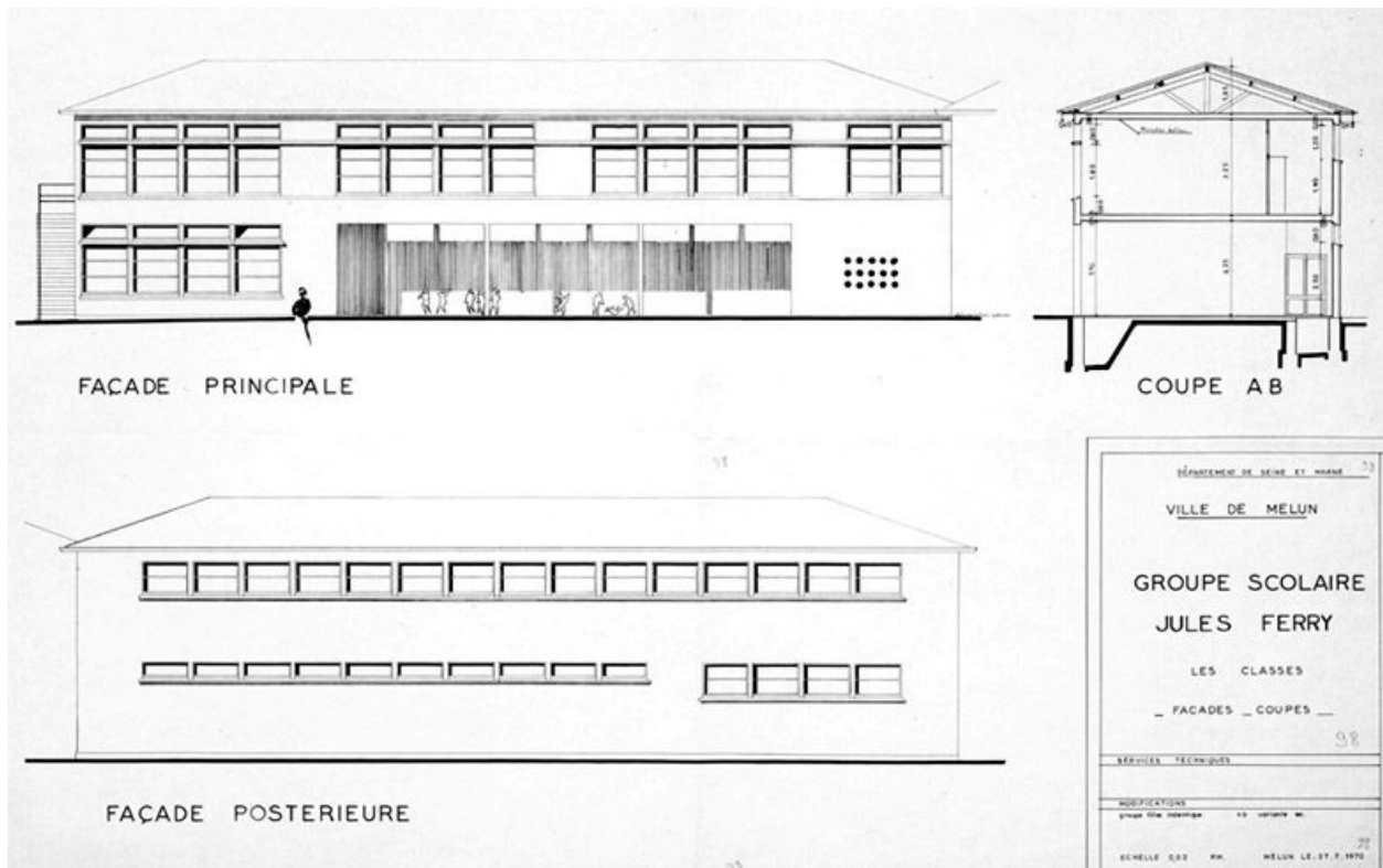
Groupe scolaire Jules-Ferry : façades et coupes. Tirage d'architecte, 1970. (AM Melun. 1 Fi 98)
