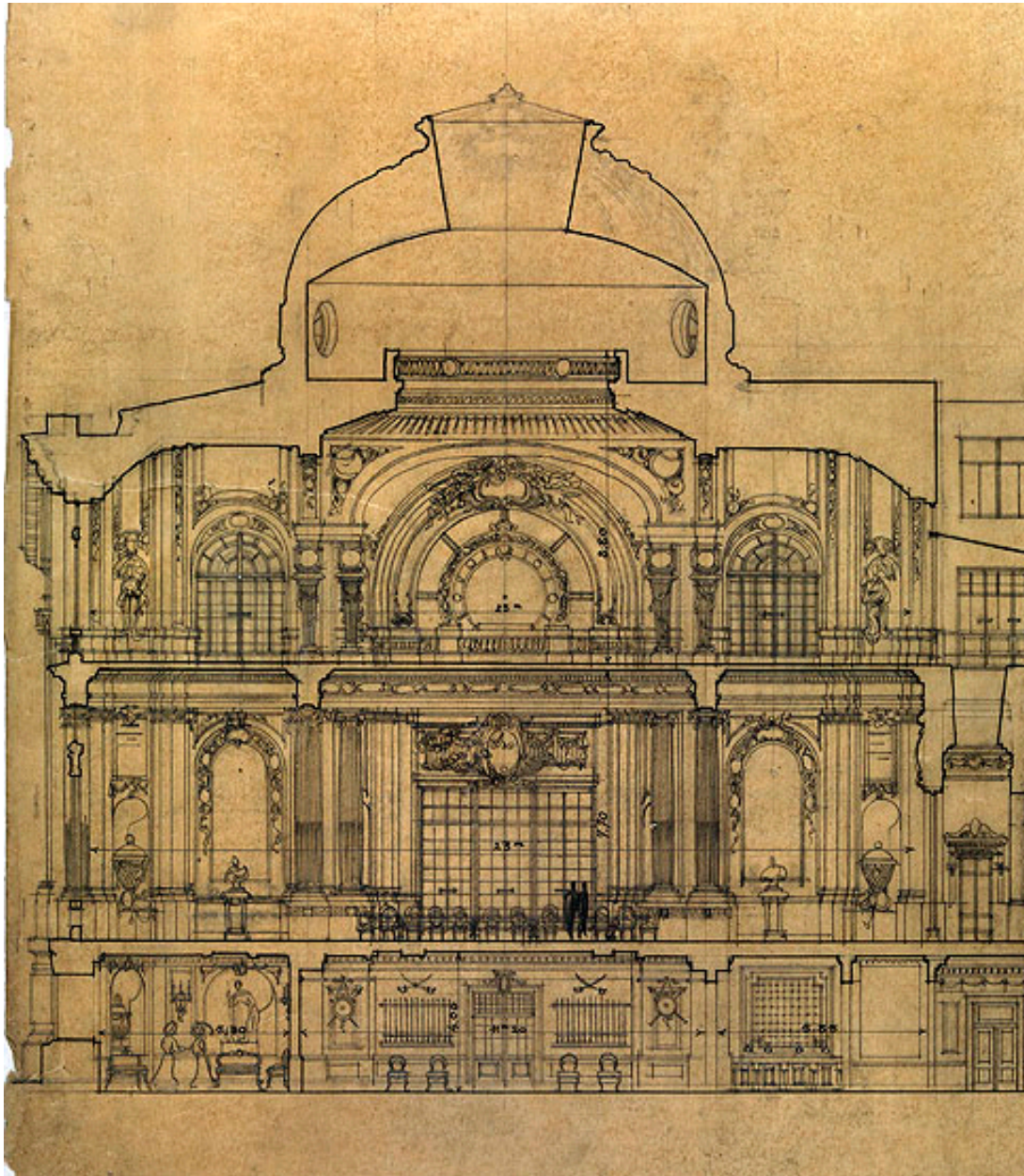
Détail de la coupe longitudinale du casino au niveau du Cercle. Dessin sur calque, 1908. (Institut français d'architecture, Fonds Guilbert Albert)
