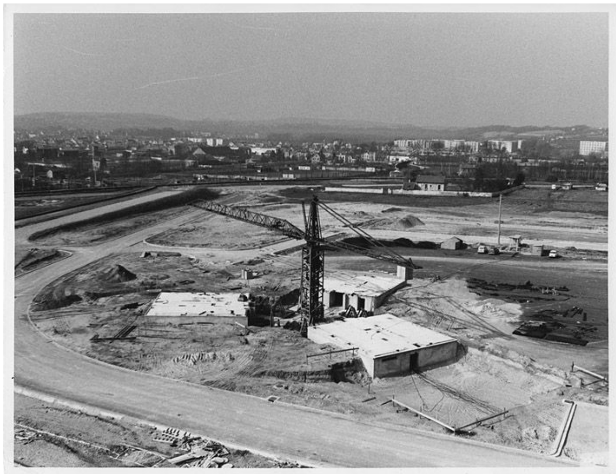
Début du chantier de construction d'une des tours de Meaux-Beauval. (OPAC Meaux)
