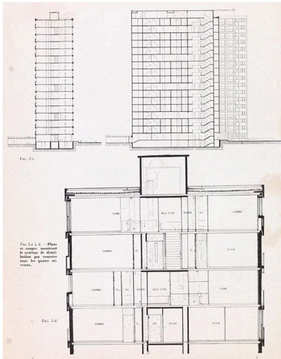
Plans et coupes montrant le système de distribution des coursives tous les 4 niveaux. (Cité de l'architecture et du patrimoine. fonds DAU 173/1)
