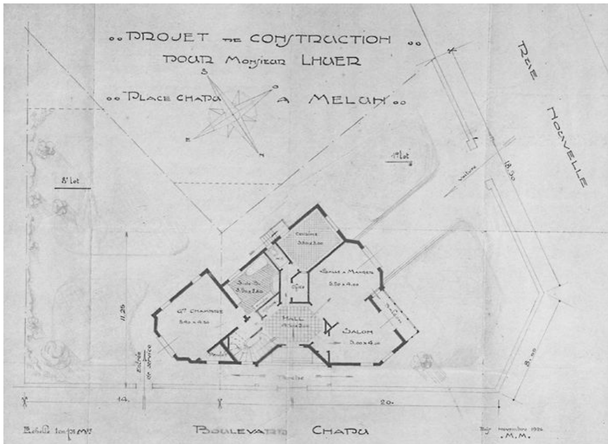
Projet de construction pour M. Lhuer place Chapu à Melun. Bleu, novembre 1926. (AM Melun. 1 Fi 606)
