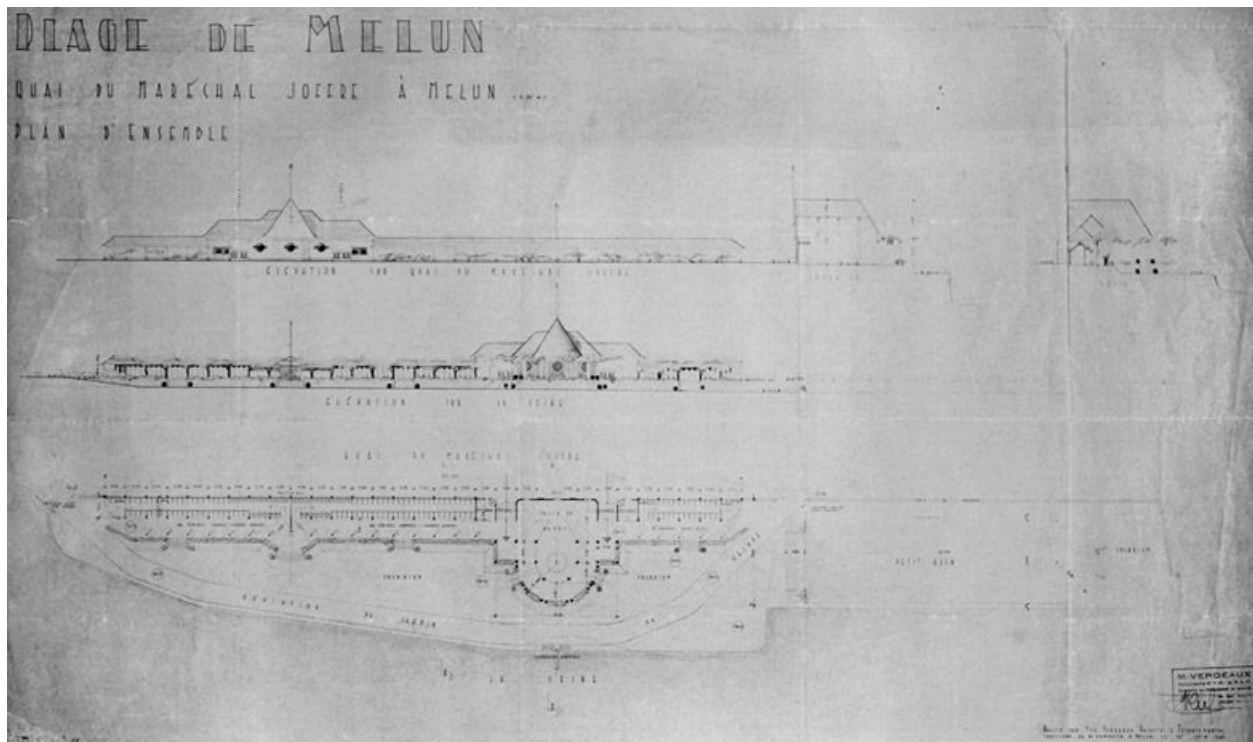
Plage de Melun. Quai du Maréchal Joffre à Melun. Plan d'ensemble. Papier, tirage d'architecte, 1942. (AM Melun. 1 Fi 1345)
