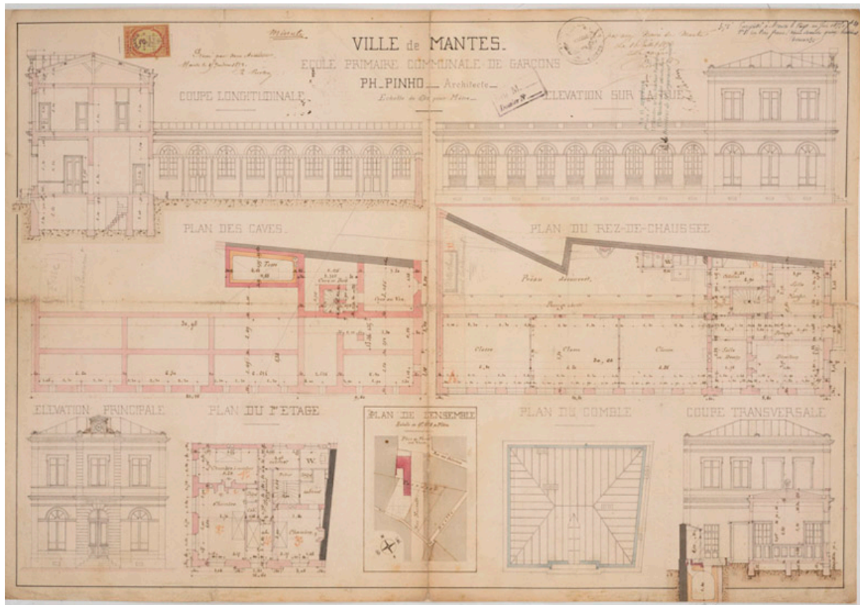
Plans et élévations de l'école. Dessins de Ph. Pinho, architecte, 1873 (AM Mantes-la-Jolie, F12 64)
