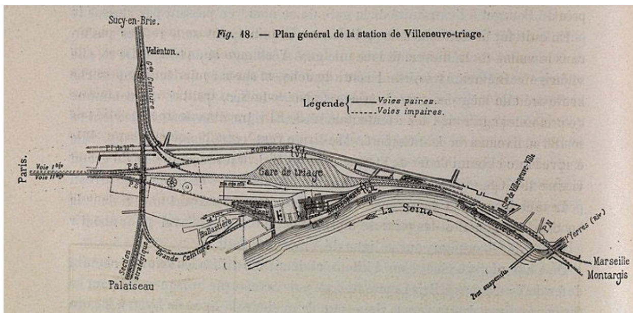
Villeneuve-Saint-Georges, gare de Villeneuve-Triage. Plan général de la station. Tiré de : Revue Générale des Chemins de Fer ", août 1885, p. 84.
