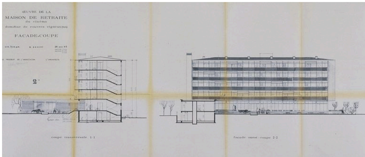
Coupe transversale et façade ouest. (AD Essonne, 1502 W 842)
