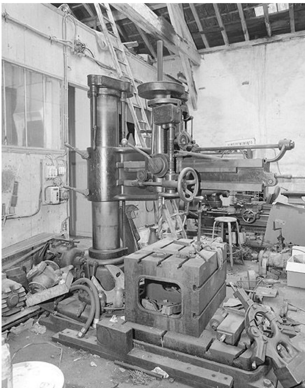
Perceuse Somua.
