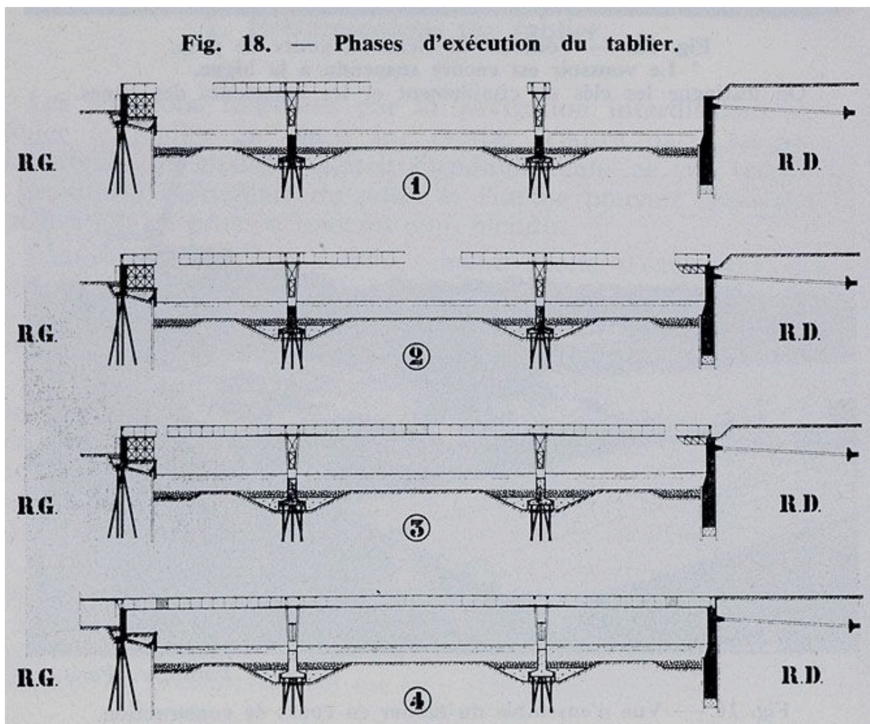
Choisy-le-Roi. Pont de Choisy (n°2). Schémas expliquant les phases successives de construction du tablier. Tiré de : Travaux, janvier 1966, n° 372.
