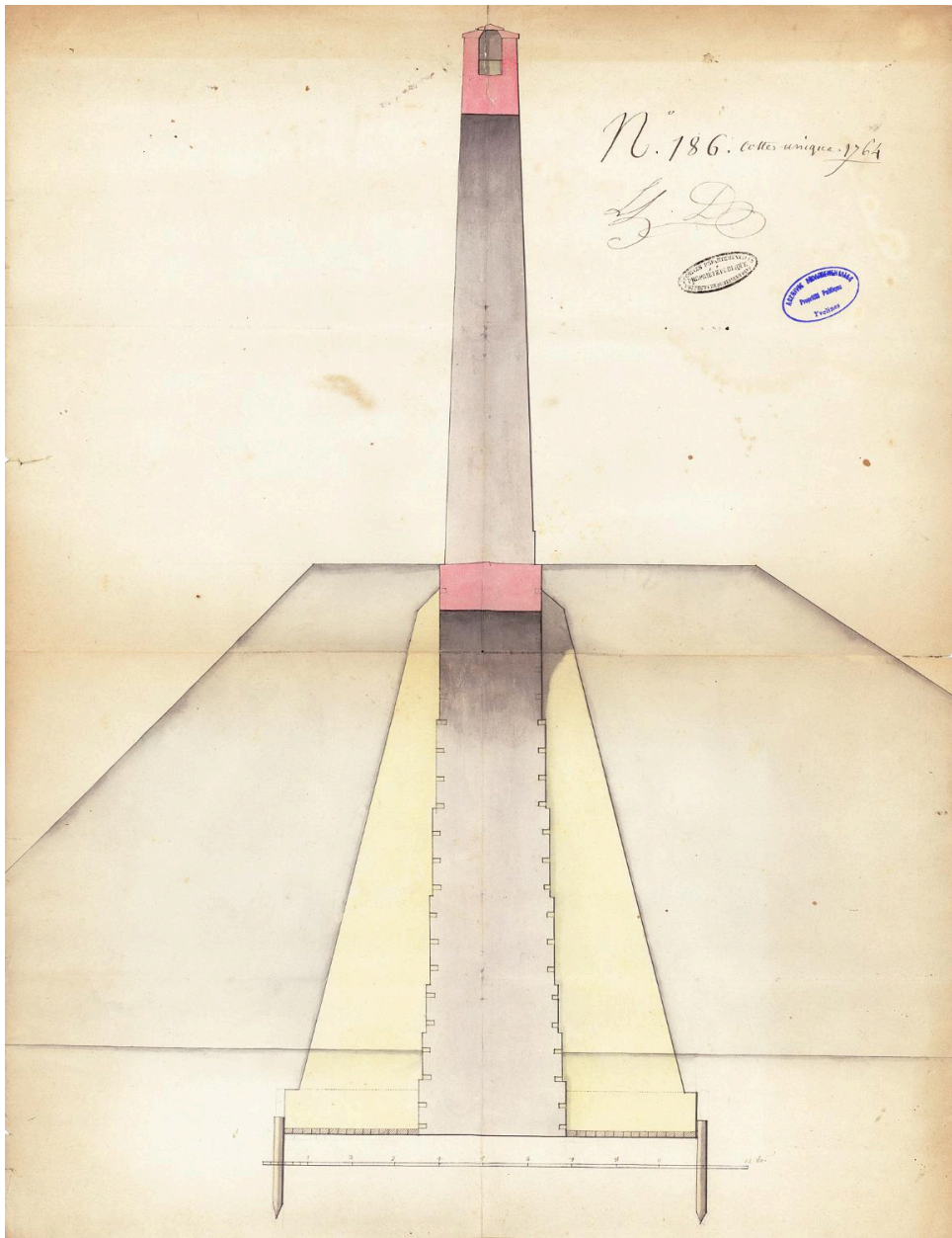
Coupe de l'aqueduc.
