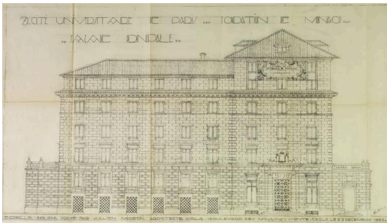
Façade principale ; Julien Médecin, architecte ; dessin, 22 décembre 1932 ; AN, 20090013/352.
