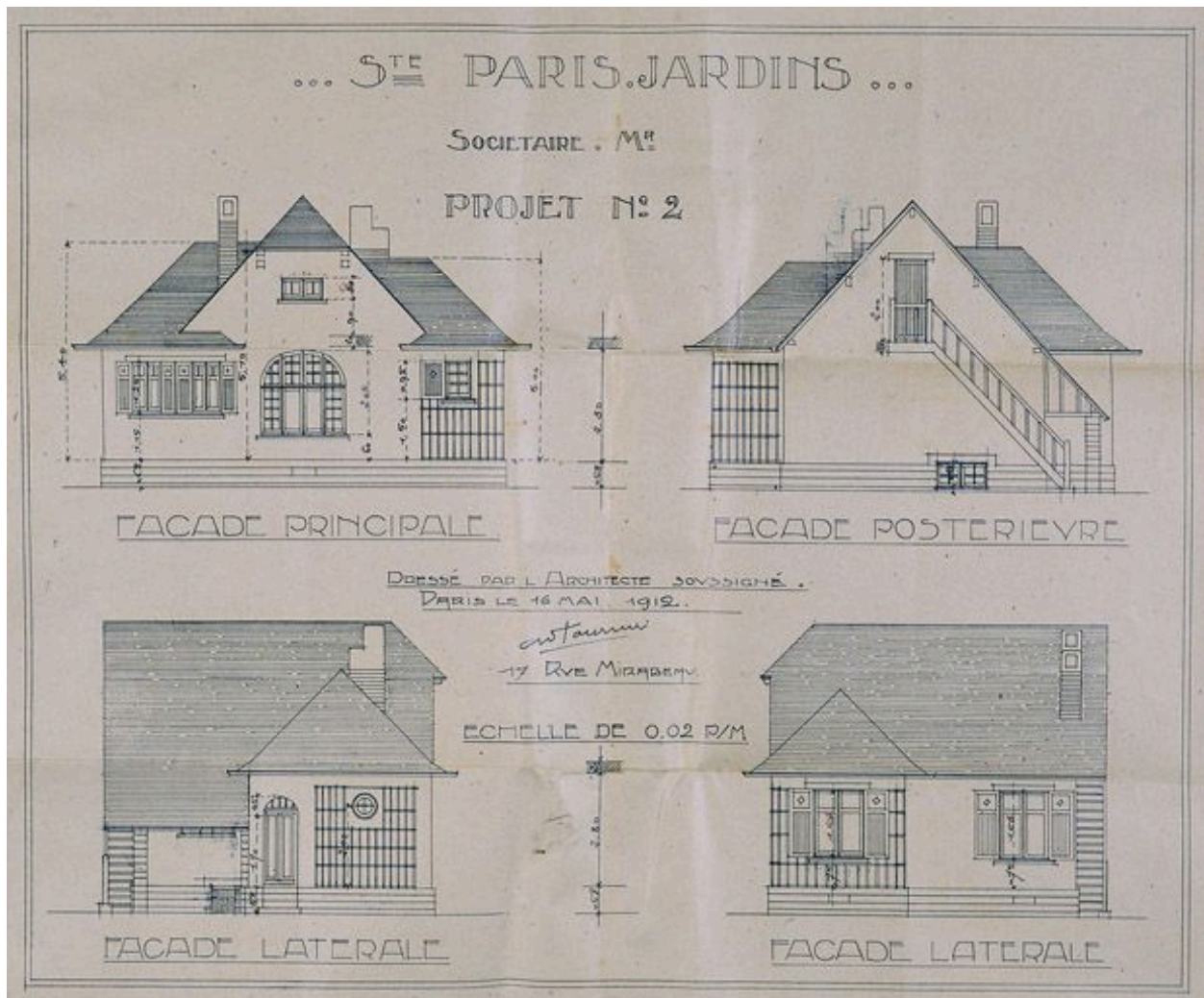
Elévations (projet n°2). (Société coopérative "Paris-Jardins" de Draveil, dossier 138)
