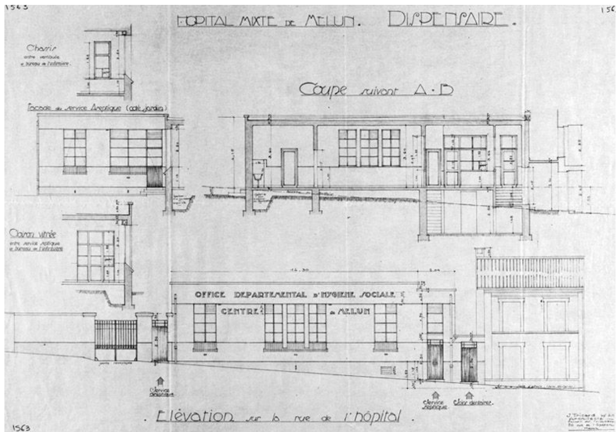
Hôpital mixte de Melun : dispensaire. Elévation sur la rue de l'Hôpital, coupe longitudinale, façade du service aseptique (côté jardin). Papier, tirage d'architecte, 1937. (AM Melun. 1 Fi 1563)
