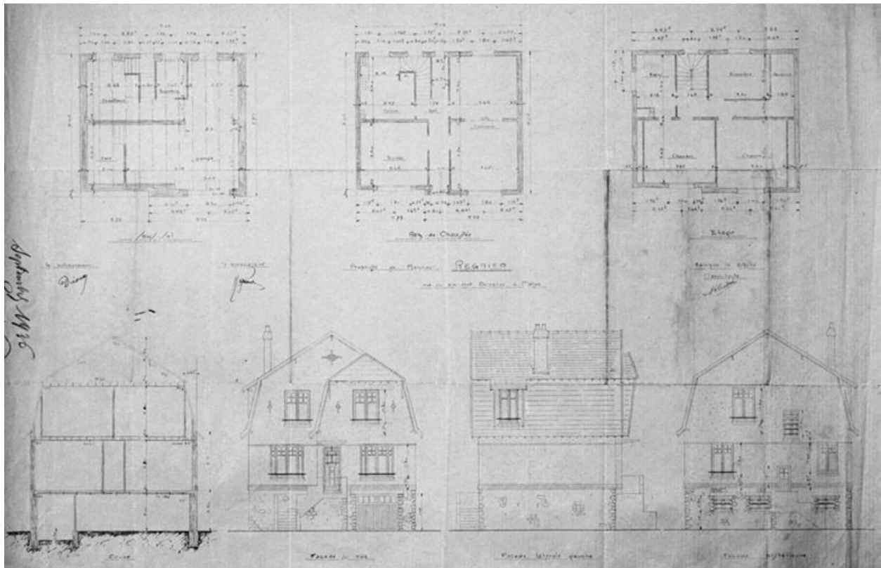
Projet de R. Leroux, architecte à Barbizon, pour la propriété de M. Régnier. Ce projet correspond au pavillon n° 33, rue du Président-Despatys (Fig.1). Tirage d'architecte, 1936 (2 mai). (AM Melun. 1 Fi 1271)
