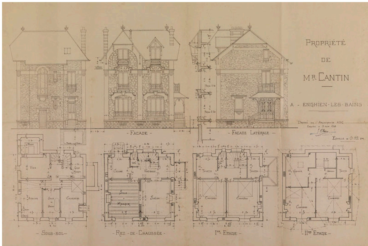
Elévations, plans d'une maison construite en 1908 pour monsieur Cantin (non localisée). (AM Enghien-les-Bains, Fonds des autorisations de permis de construire)
