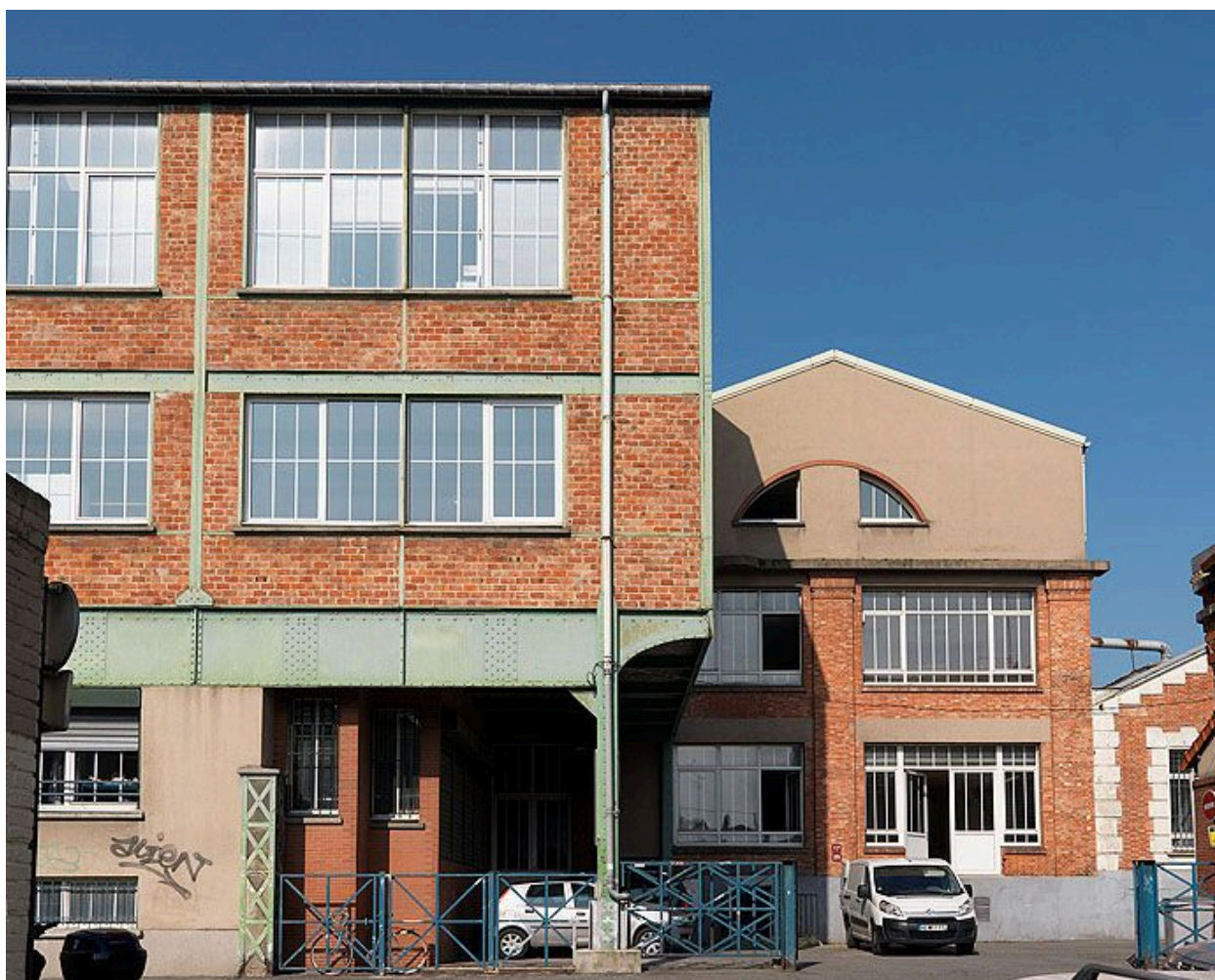
93, Bagnole, biscuiterie Belin , 15-17 rue Charles-Graindorge. Détail des appareils de brique pleine et creuse et du pan de fer du mur de façade des locaux de production.
