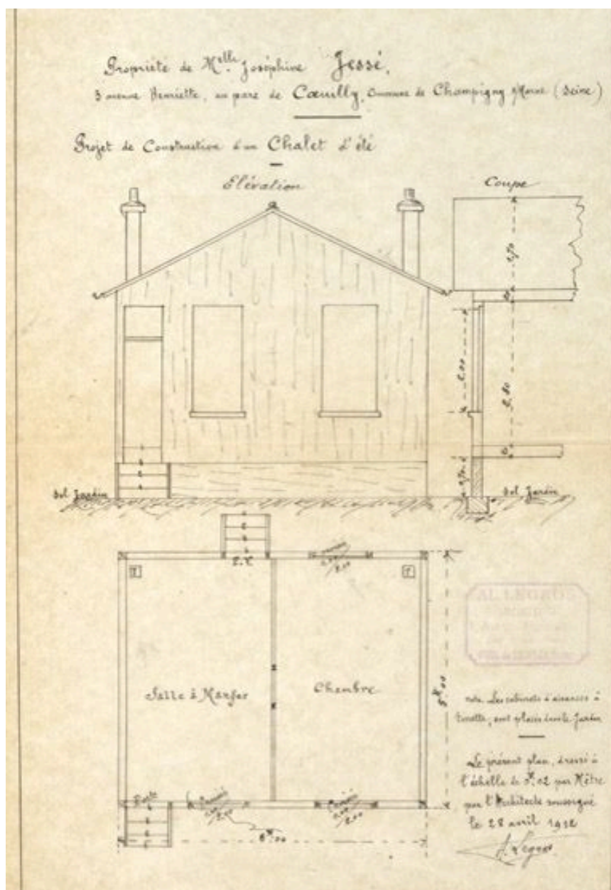
Projet de construction d'un chalet d'été, 3 avenue Henriette. Plan et élévation, 1912. Legros, Adolphe (architecte). (AM Champigny-sur-Marne. Boîte 008 838)
