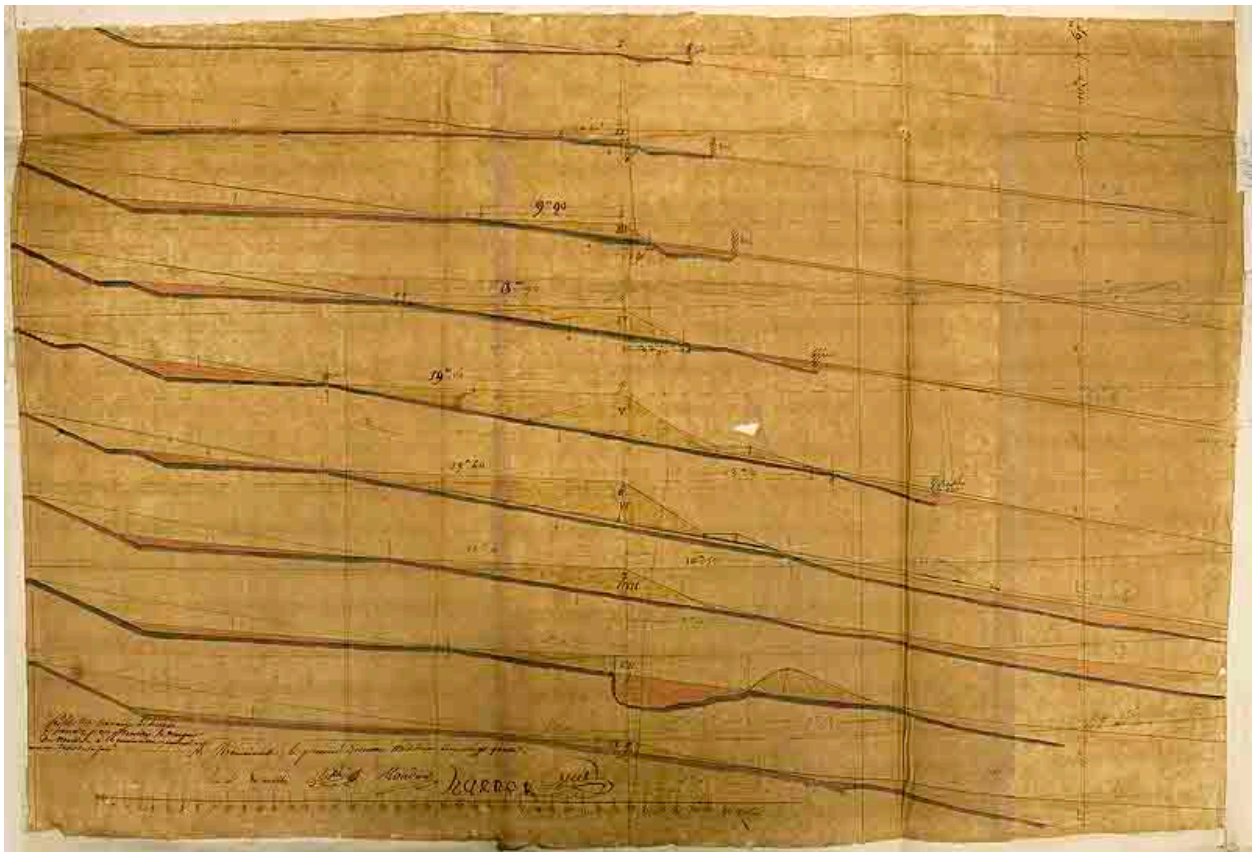
Dessin, projet de terrassement pour le parc du château? (Ecole nationale des ponts et chaussées, Champs-sur-Marne. Fonds Charles-François Mandar)
