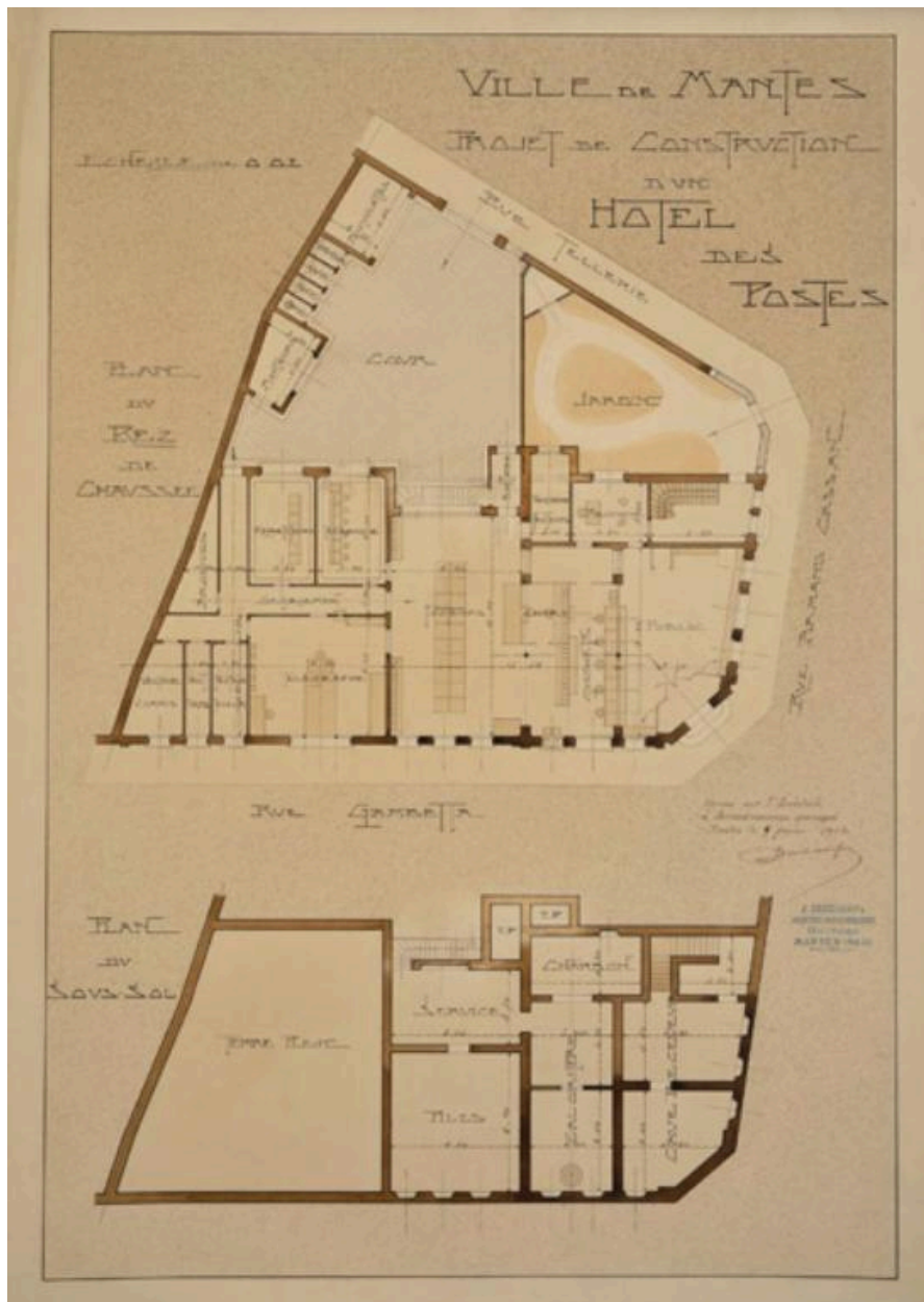
Plan du rez-de-chaussée et du sous-sol. Dessin de J. Deschamps. 1912. (AM Mantes-la-Jolie, Fi 162)
