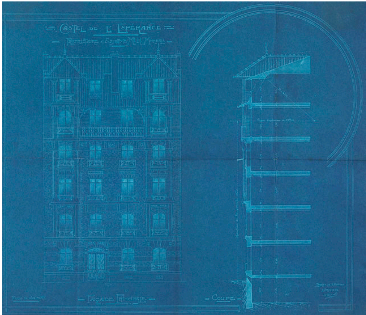
Elévation et coupe de l'immeuble donnant sur la rue Félix Faure (1911). (AM Enghien-les-Bains, 1T 97)
