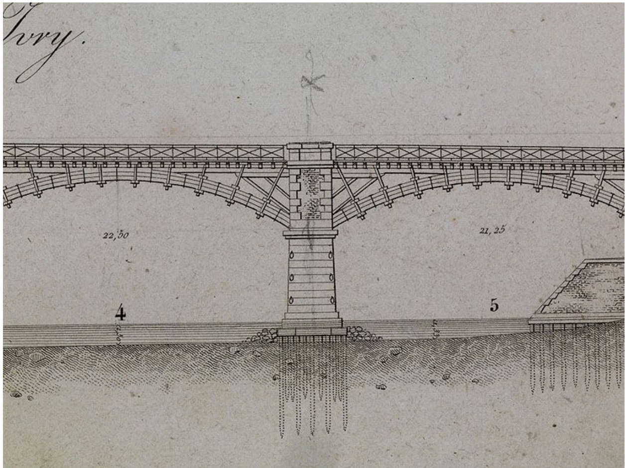
Ivry-sur-Seine. Pont d'Ivry (n°1). Détail de l'élévation d'une pile en rivière et de deux arches. Tiré de : Pont d'Ivry en bois, sur piles en pierre, traversant la Seine... / MHC Emmery. Paris : Carilian-Goeury, 1832. (Ecole nationale des ponts et chaussées)
