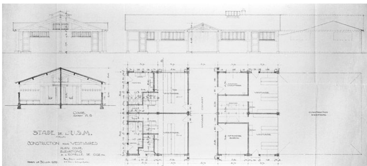
Stade de l'USM : projet de vestiaires. Tirage d'architecte, 1939. (AM Melun. 1 Fi 1388)
