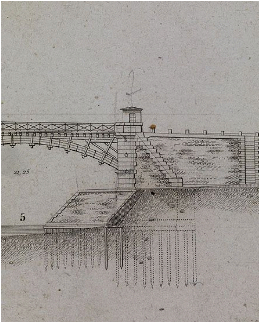
Ivry-sur-Seine. Pont d'Ivry (n°1). Détail de l'élévation d'une culée. Tiré de : Pont d'Ivry en bois, sur piles en pierre, traversant la Seine... / MHC Emmery. Paris : Carilian-Goeury, 1832. (Ecole nationale des ponts et chaussées)
