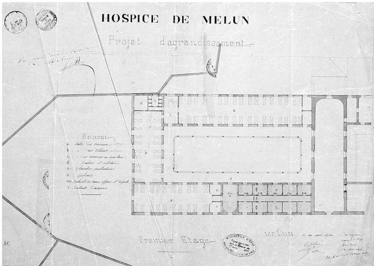
Hospice de Melun, projet d'agrandissement : plan du premier étage. Calque sur toile aquarellé, 20 mai 1854. (BM Melun. II 10)
