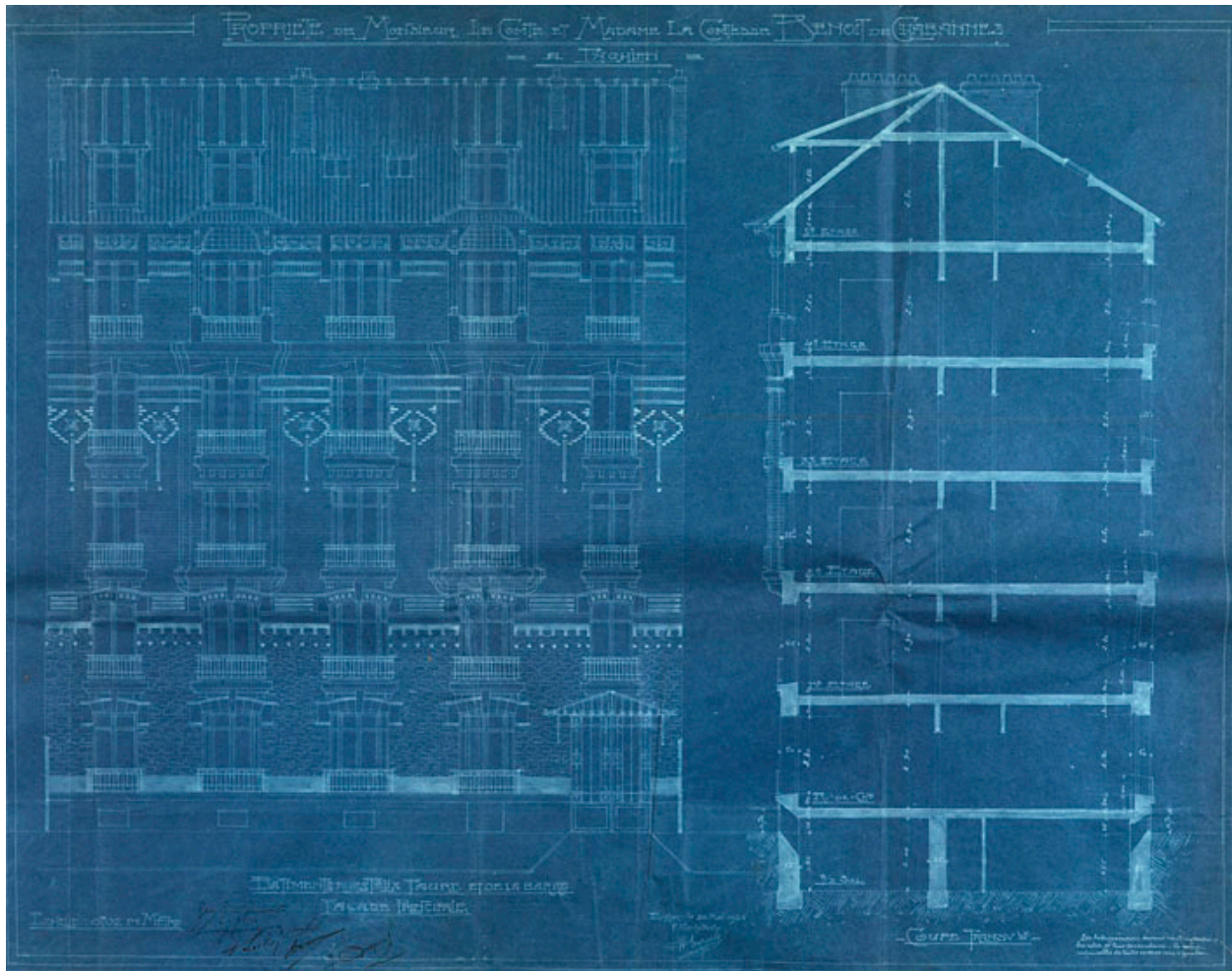
Coupe et élévation de l'un des immeubles du lotissement. (AM Enghien-les-Bains, Fonds des autorisations de permis de construire)
