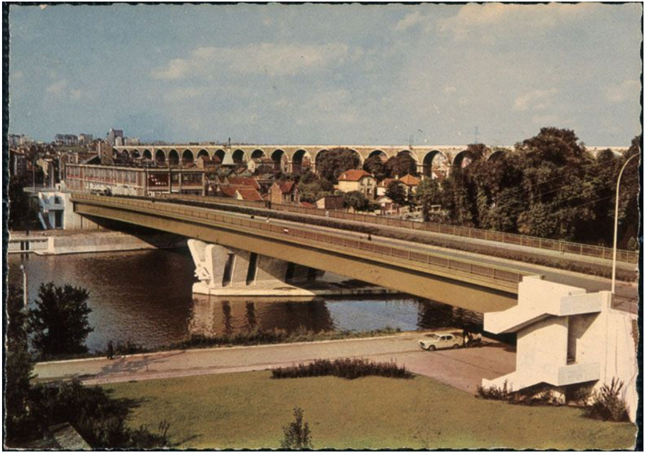
Le nouveau pont de Nogent dessiné par Paul Domenc (architecte), au second plan, le viaduc de Nogent. Carte postale. (AD Val-de-Marne. 2Fi Champigny 528)
