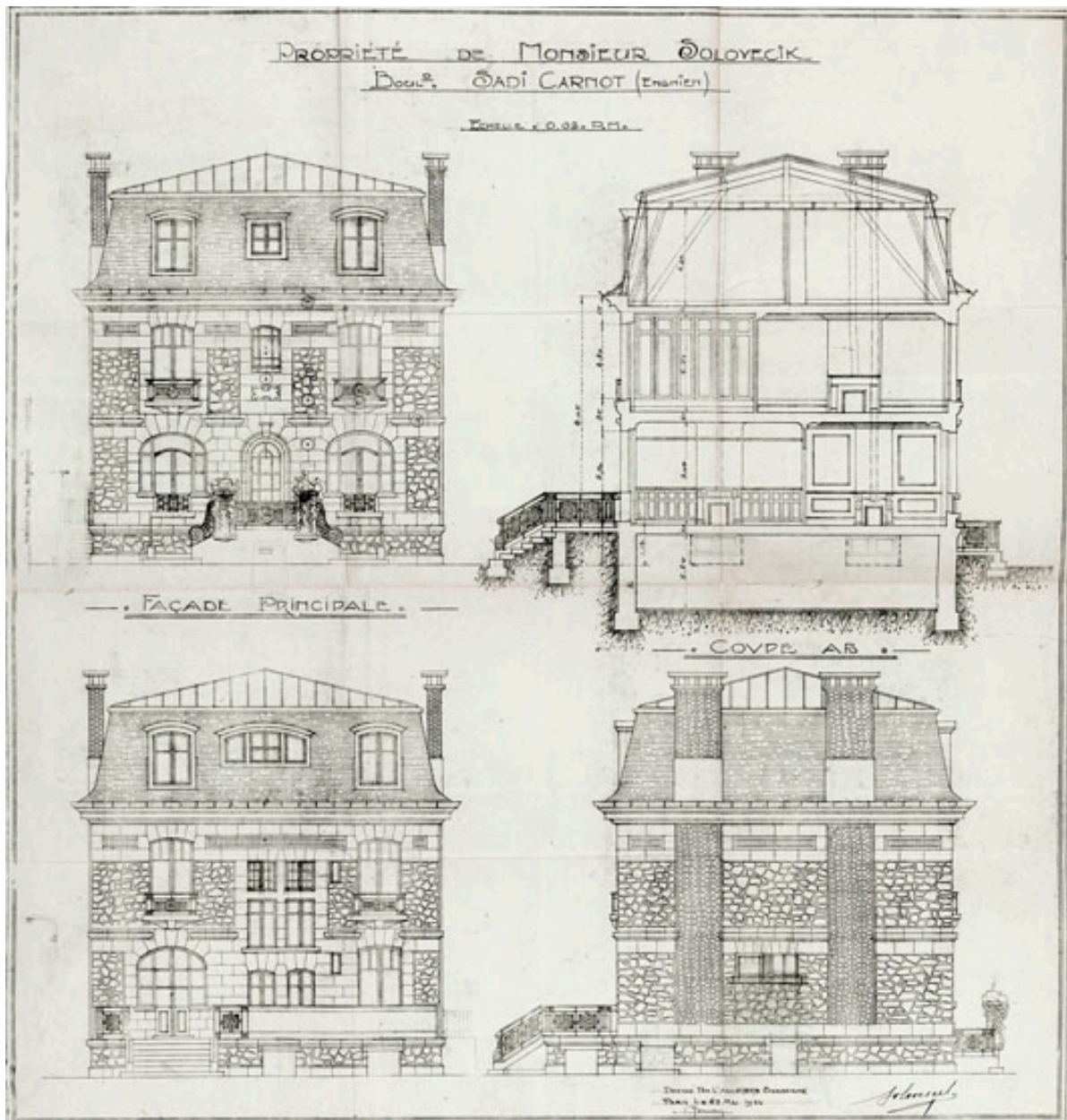
Elévations et coupe d'une maison pour monsieur Solovecik, construite en 1924, 17 boulevard Sadi Carnot. (AM Enghien-les-Bains)
