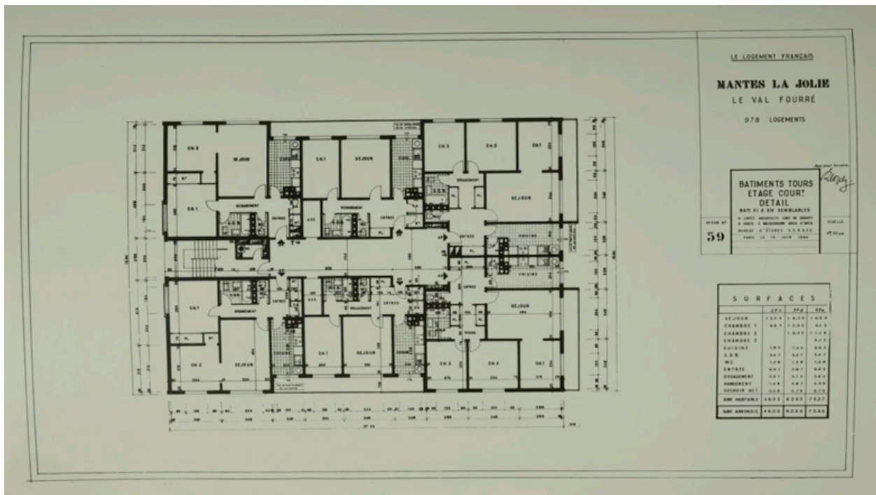
Quartier 1, des Ecrivains. Plan d'un étage courant des tours de vingt étages. (Archives Nationales, Direction de l'Habitat et de la Construction, 19840091/58-59)
