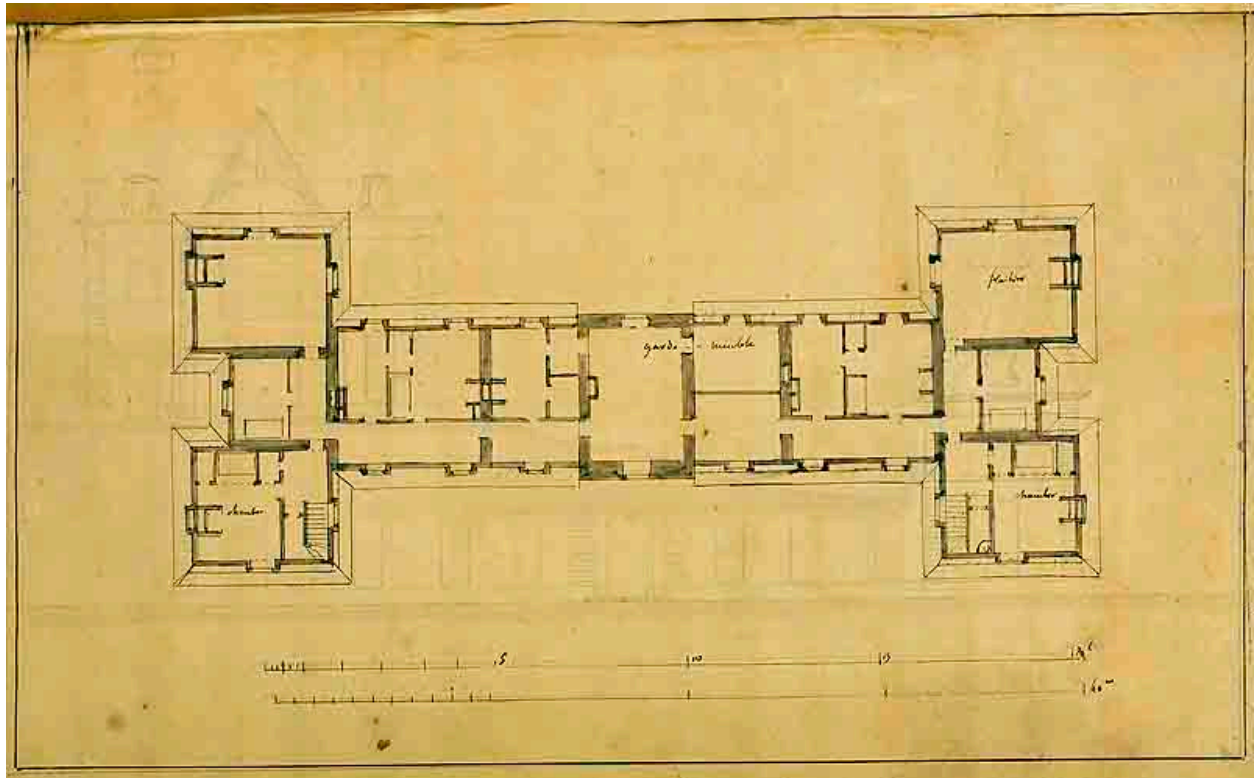
Plan du rez-de-chaussée du château. (Ecole nationale des ponts et chaussées, Champs-sur-Marne. Fonds Charles-François Mandar)
