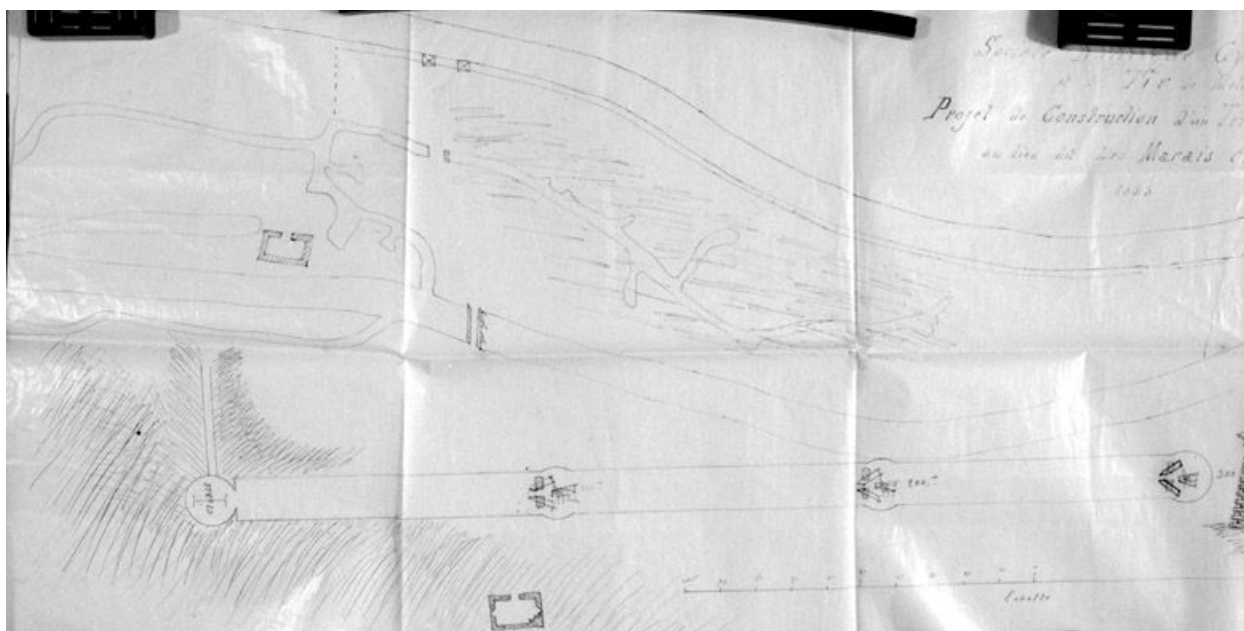
Projet pour établir un tir au fusil de 300 mètres, au lieu-dit Les Marais (en bordure de l'Almont). Détail : le plan au sol. Calque, 5 avril 1883. (AM Melun. 3 R 2)
