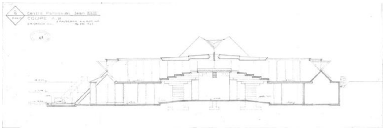
Coupe A-B.
