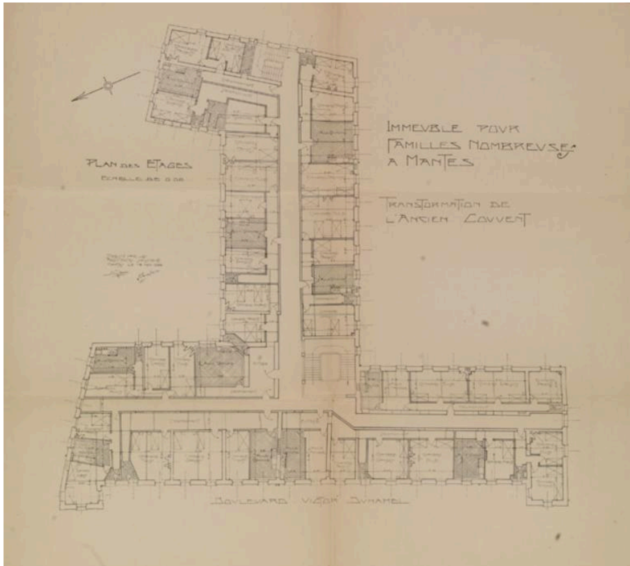
Plan type des étages de l'immeuble pour familles nombreuses, Cauzard, Marabout (architectes), 1922 (AM Mantes-la-Jolie 7M 2(2)).
