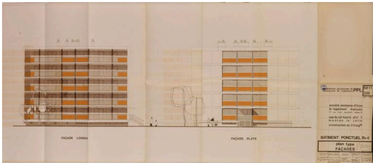
Quartier 7. Façades des bâtiments dits "ponctuels", c'est-à-dire des immeubles plots. 1968. Mantes-la-Jolie. Permis de construire 44/68.
