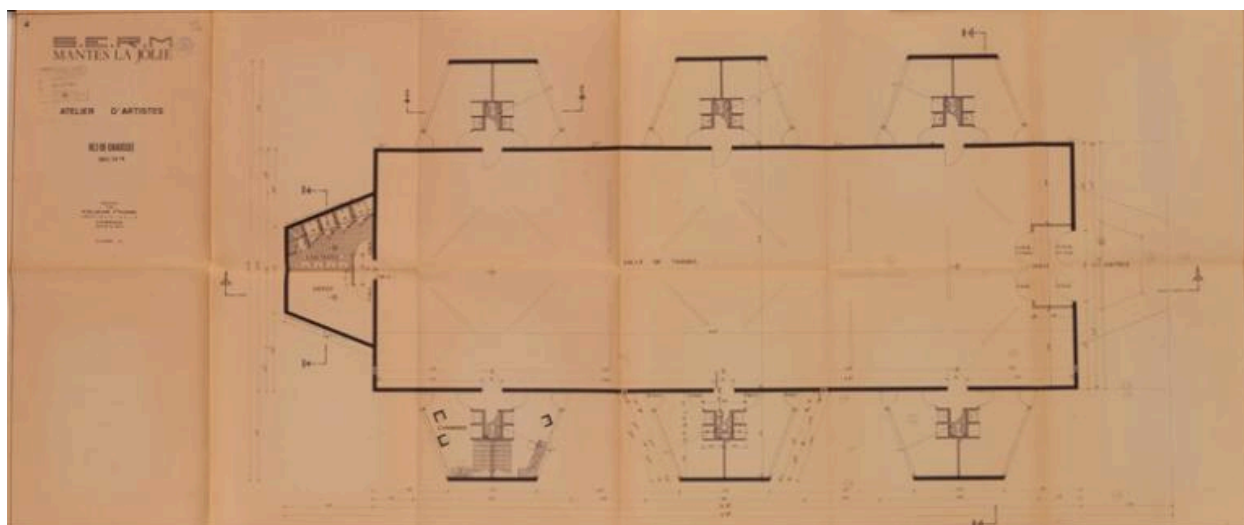
Quartier 7, 7 bis et village d'artistes. Plan du rez-de-chaussée de l'atelier collectif (non réalisé). Projet de 1968. Mantes-la-Jolie. Permis de construire 21-35/67.
