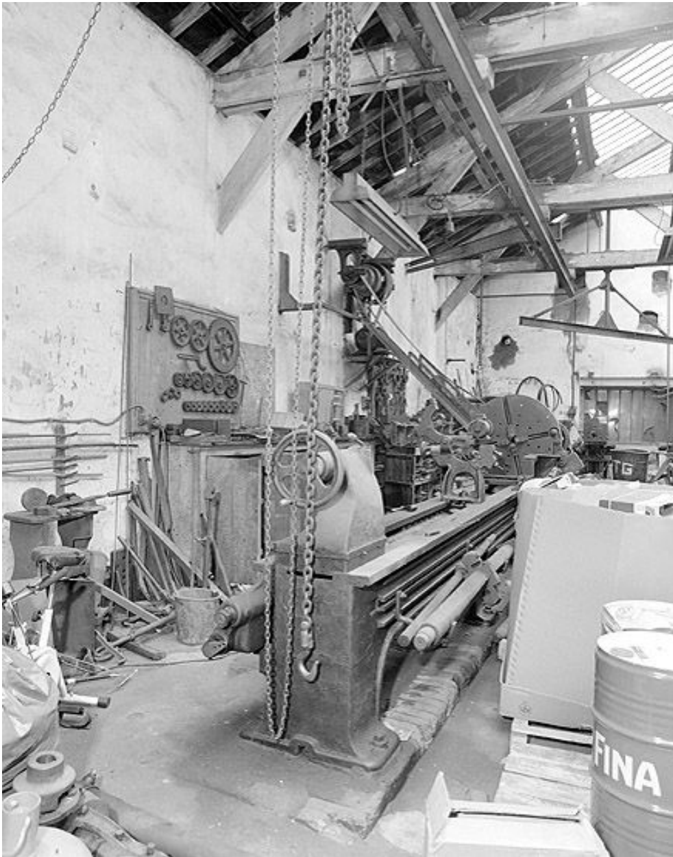
Grand tour avec moteur annexe et courroie de transmission pour fabrication d'arbres d'hélices : vue générale.
