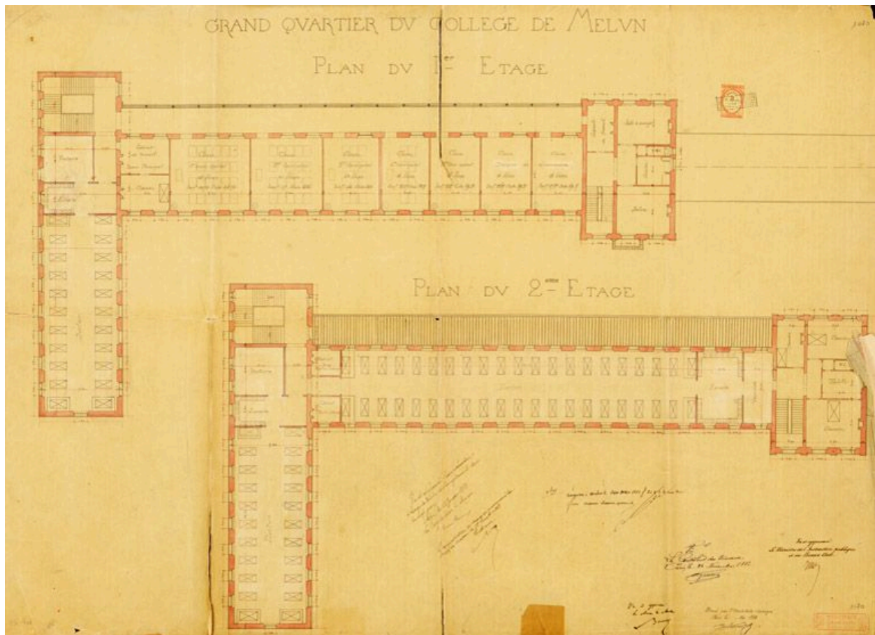
Grand quartier du collège de Melun : plan du premier et du deuxième étages, 1882. (AM Melun. 1 Fi 1070)
