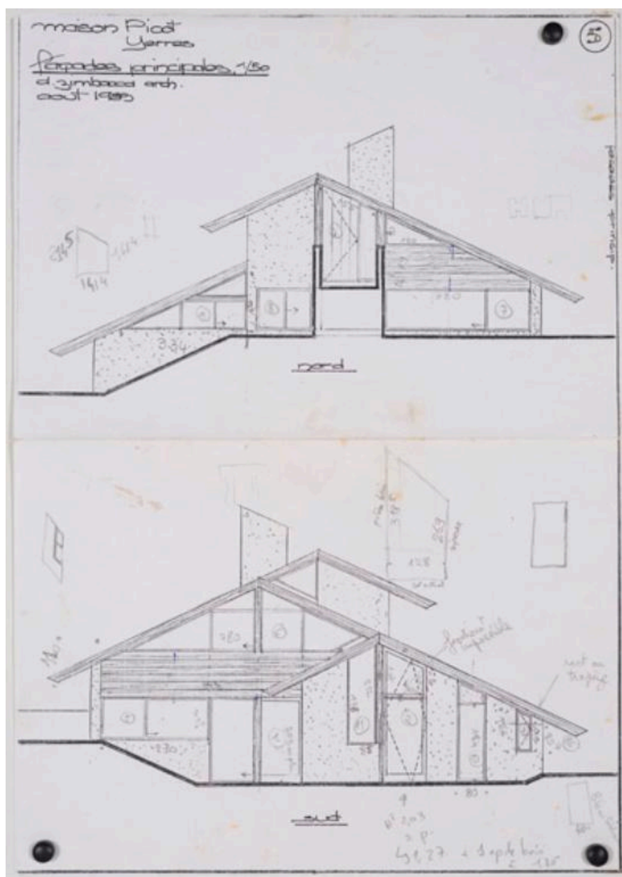
Coupe de la maison Picot, Hameau de Bellevue, Yerres, 1989.
