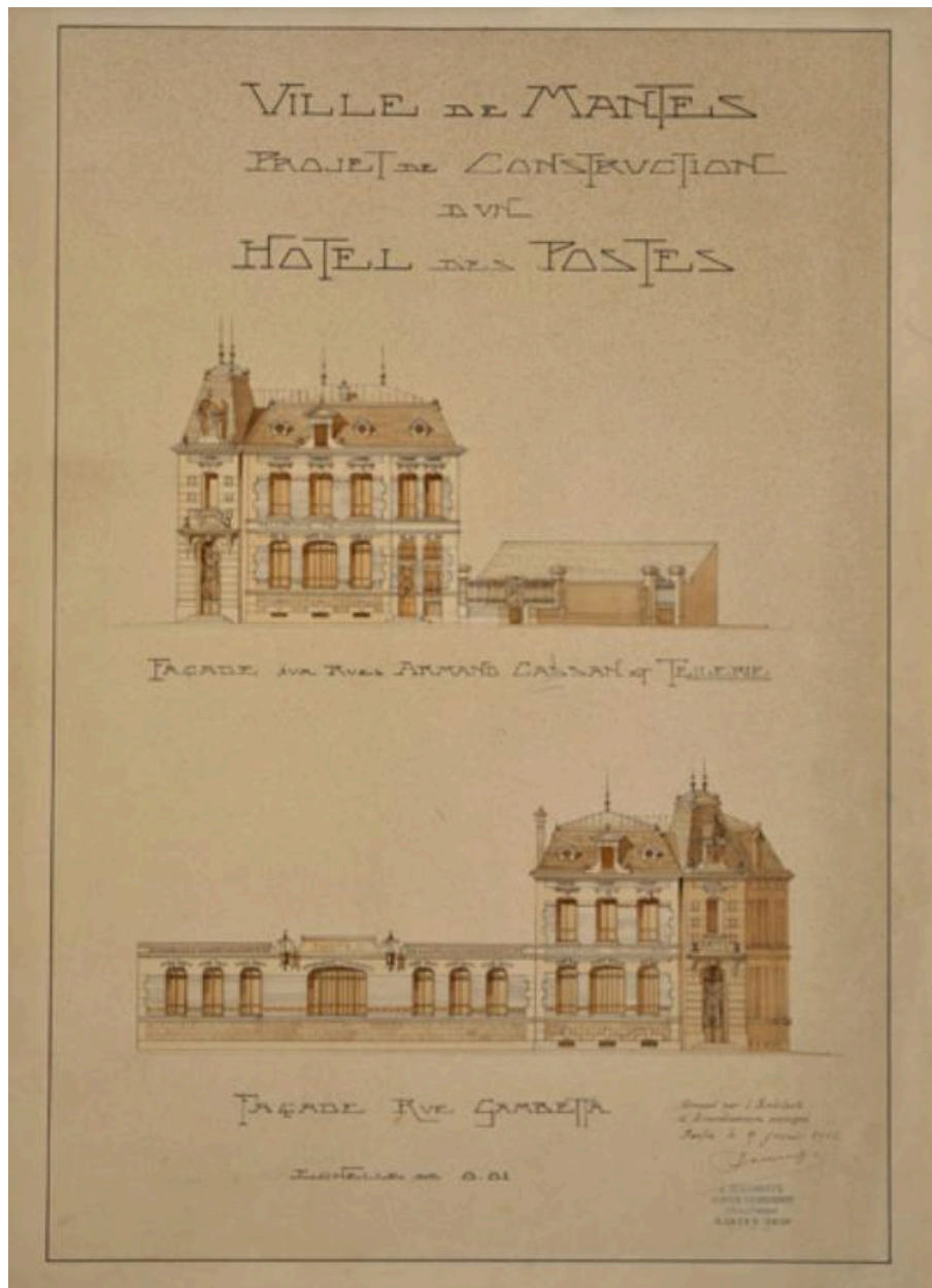
Façades sur rue. Dessins de J. Deschamps. 1912. (AM Mantes-la-Jolie, Fi 160)
