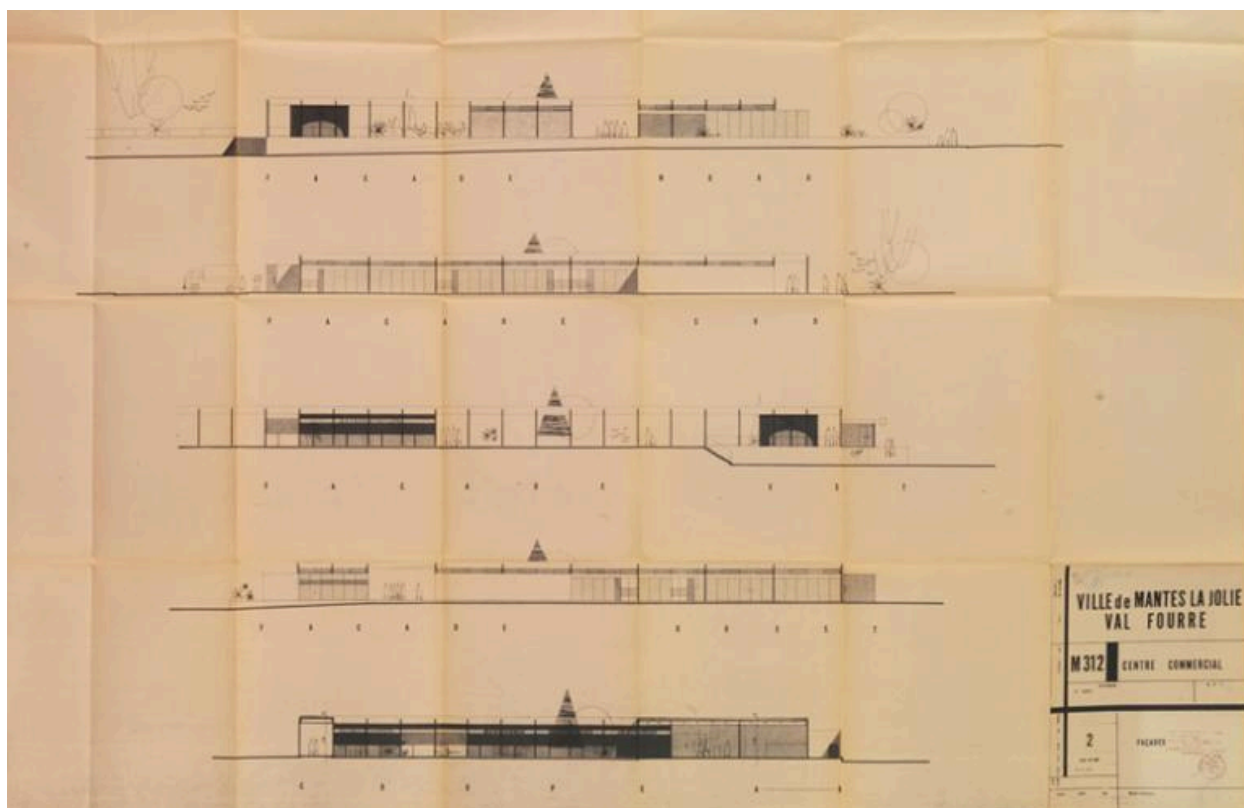
Quartier 2. Projet de centre commercial. 1963. Mantes-la-Jolie. Permis de construire 94/63.
